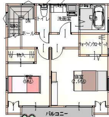
2階 平面図 S:1/100
