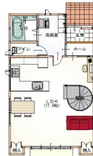
1階 平面図 S:1/100
