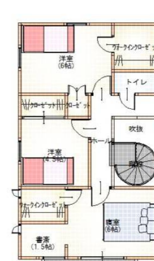
2階 平面図 S:1/100
