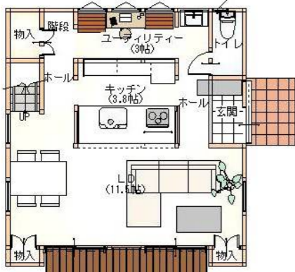
1階 平面図 S:1/100
