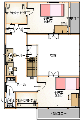
2階 平面図 S:1/100
