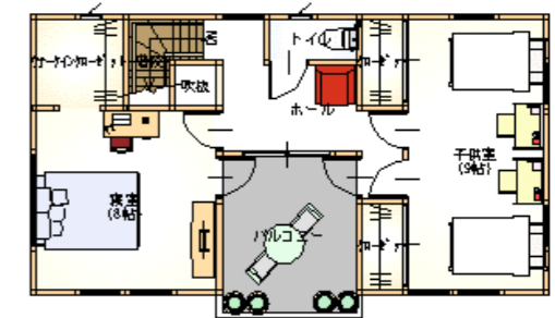
2階 平面図 S:1/100
