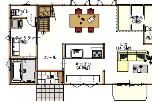
1階 平面図 S:1/100
