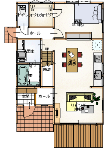
1階 平面図 S:1/100
