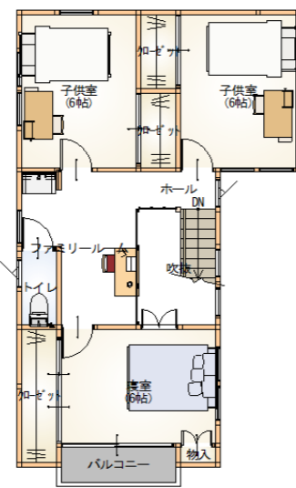
2階 平面図 S:1/100
