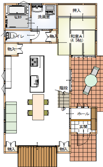
1階 平面図 S:1/100
