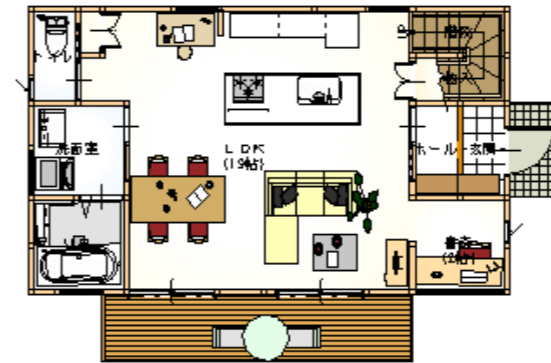
1階 平面図 S:1/100
